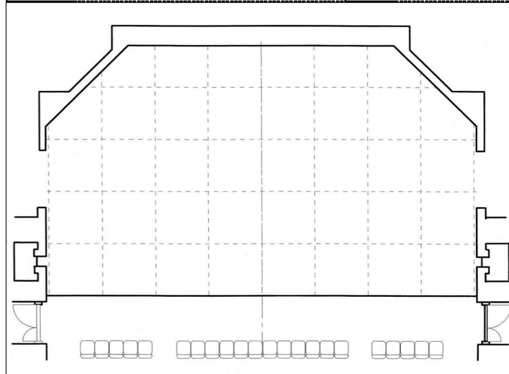
舞台概要: 間口14.59m(開口部), 9m(最奥部) 奥行5.86m~8.64m(上手・下手から各約1間半) 緞帳22秒 スクリーン35秒
